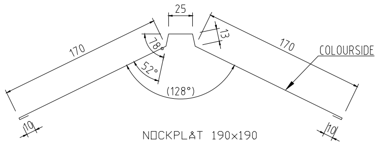
NOCKPLÅT 190x190 Tj=0,5-0,6 L=2000mm KB=410mm
