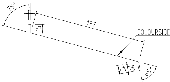
UNDERBLECK FÄNSTER 190 Tj=0,6 L=1200, 1500, 2000mm KB=241mm
