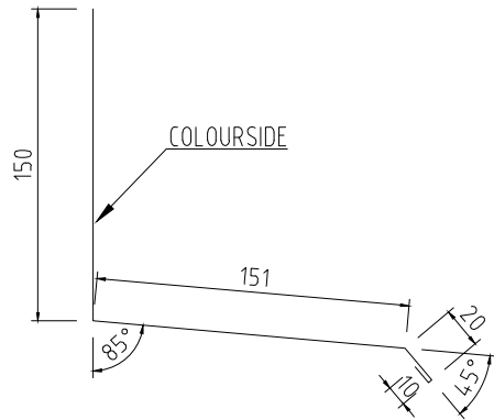
STÅNDSKIVA 170x150 Tj=0,5-0,6 L=2000mm KB=331mm
