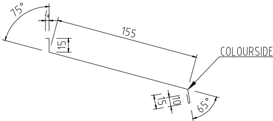
UNDERBLECK FÄNSTER 150 Tj=0,6 L=1200, 1500, 2000mm KB=199mm
