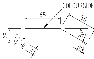
GAVELBESLAG KNÄCKT 25x65x55 Tj=0,5-0,6 L=2000mm KB=177mm
