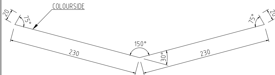
RÄNNDALEPLÅT RAK 230x230 Tj=0,5-0,6 L=2000mm KB=500mm
