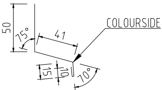
ÖVERBLECK FÄNSTER 40 Tj=0,6 L=1200, 1500, 2000mm KB=116mm
