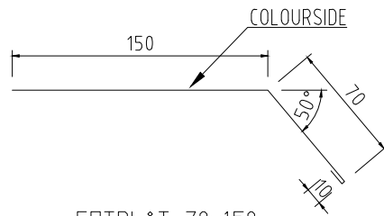
FÖTPLÅT 70x150 Tj=0,5-0,6 L=2000mm KB=230mm
