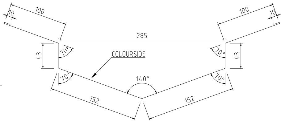
RÄNNDALEPLÅT KNÄCKT 152x152 Tj=0,5-0,6 L=2000mm KB=610mm
