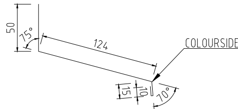
ÖVERBLECK FÄNSTER 120 Tj=0,6 L=1200, 1500, 2000mm KB=199mm
