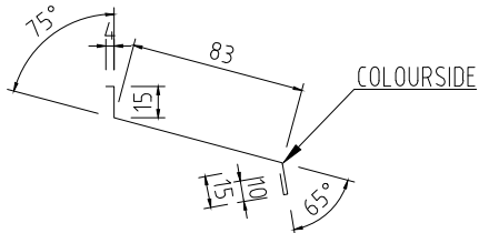
UNDERBLECK FÄNSTER 80 Tj=0,6 L=1200, 1500, 2000mm KB=127mm
