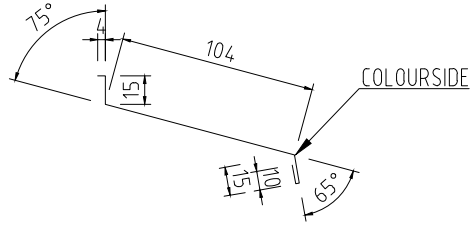
UNDERBLECK FÄNSTER 100 Tj=0,6 L=1200, 1500, 2000mm KB=148mm
