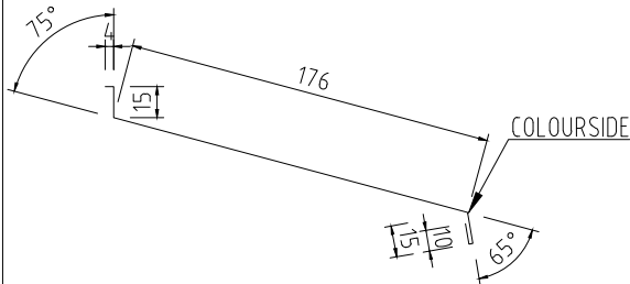
UNDERBLECK FÄNSTER 170 Tj=0,6 L=1200, 1500, 2000mm KB=220mm
