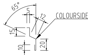
TRÄSKELBLECK 1230 Tj=0,5-0,6 L=1230mm KB=62mm
