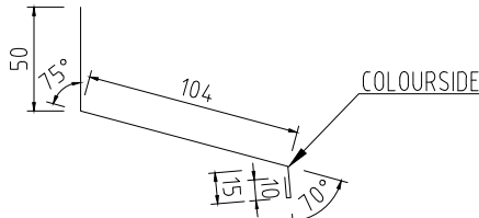
ÖVERBLECK FÄNSTER 100 Tj=0,6 L=1200, 1500, 2000mm KB=179mm
