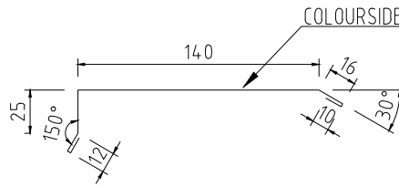
GAVELBESLAG RAK 25x140 Tj=0,5-0,6 L=2000mm KB=213mm
