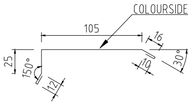
GAVELBESLAG RAK 25x105 Tj=0,5-0,6 L=2000mm KB=178mm
