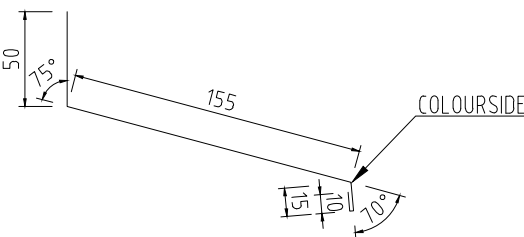
ÖVERBLECK FÄNSTER 150 Tj=0,6 L=1200, 1500, 2000mm KB=230mm
