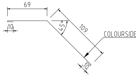
FÖTPLÅT 69x109 VÄNDBAR Tj=0,5-0,6 L=2000mm KB=198mm
