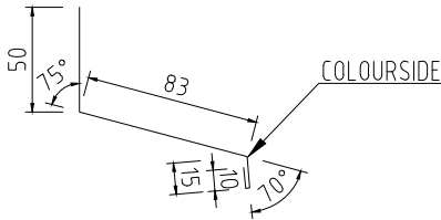
ÖVERBLECK FÄNSTER 80 Tj=0,6 L=1200, 1500, 2000mm KB=158mm
