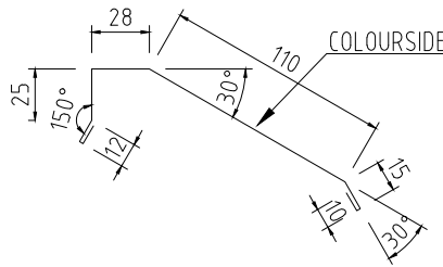
GAVELBESLAG KNÄCKT 25x28x110 Tj=0,5-0,6 L=2000mm KB=210mm
