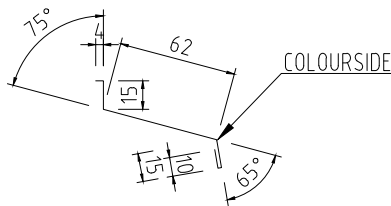
UNDERBLECK FÄNSTER 60 Tj=0,6 L=1200, 1500, 2000mm KB=106mm
