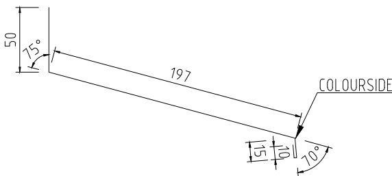
ÖVERBLECK FÄNSTER 190 Tj=0,6 L=1200, 1500, 2000mm KB=272mm
