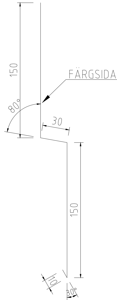
SOCKELBLECK 1 Tj=0,6 PE
