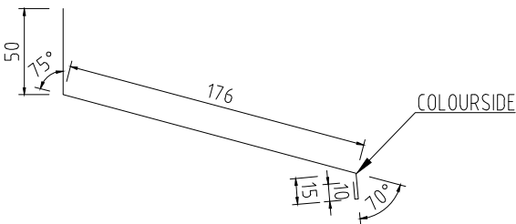
ÖVERBLECK FÄNSTER 170 Tj=0,6 L=1200, 1500, 2000mm KB=251mm
