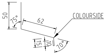
ÖVERBLECK FÄNSTER 60 Tj=0,6 L=1200, 1500, 2000mm KB=137mm
